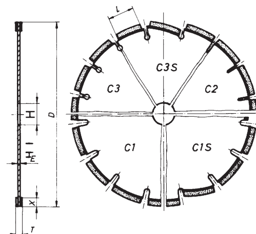
Oblika jedra diamantne krožne žage
